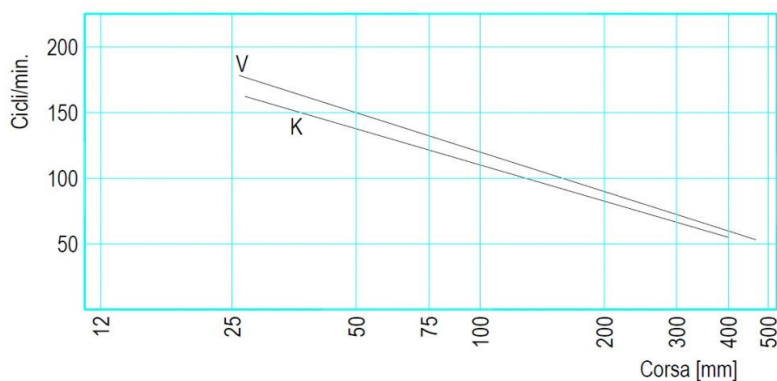
Diagramma cicli/minuto
